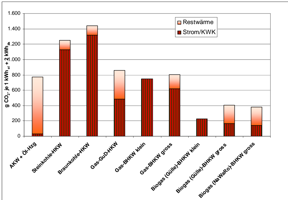
Bild 5 CO 2 -Emissionen der Strom- und Wärmeerzeugung (inkl. vorgelagerter Prozesse und Stoffeinsatz zur Anlagenherstellung) bei der „Brutto“-Betrachtung; Restwärme aus Öl-Heizung
