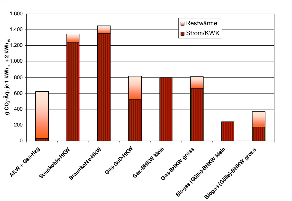
Bild 6 Gesamte Treibhausgas-Emissionen der Strom- und Wärmeerzeugung (inkl. vorgelagerter Prozesse und Stoffeinsatz zur Anlagenherstellung) bei der „Brutto“-Betrachtung; Restwärme aus Gas-Heizung
