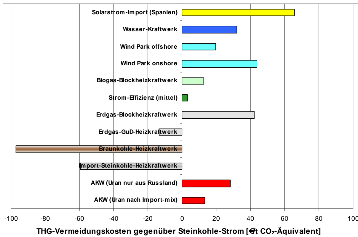
Bild 7 Spezifische Treibhausgas-Vermeidungskosten für ausgewählte Stromsysteme
