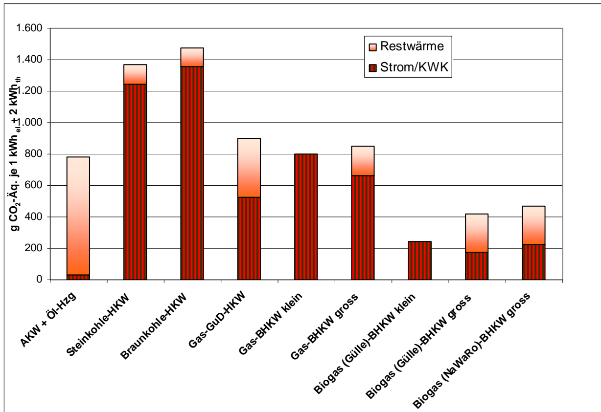
Bild 4 Gesamte Treibhausgas-Emissionen der Strom- und Wärmeerzeugung (inkl. vorgelagerter Prozesse und Stoffeinsatz zur Anlagenherstellung) bei der „Brutto“-Betrachtung; Restwärme aus Öl-Heizung
