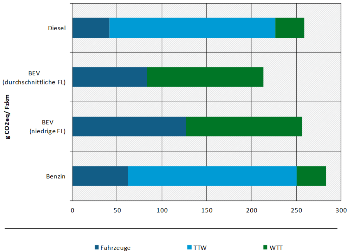
Abbildung 9: Treibhausgasemissionen eines mittleren Pkw im Antriebsvergleich (Status quo-Betrachtung mit heutigem deutschen Strommix)
